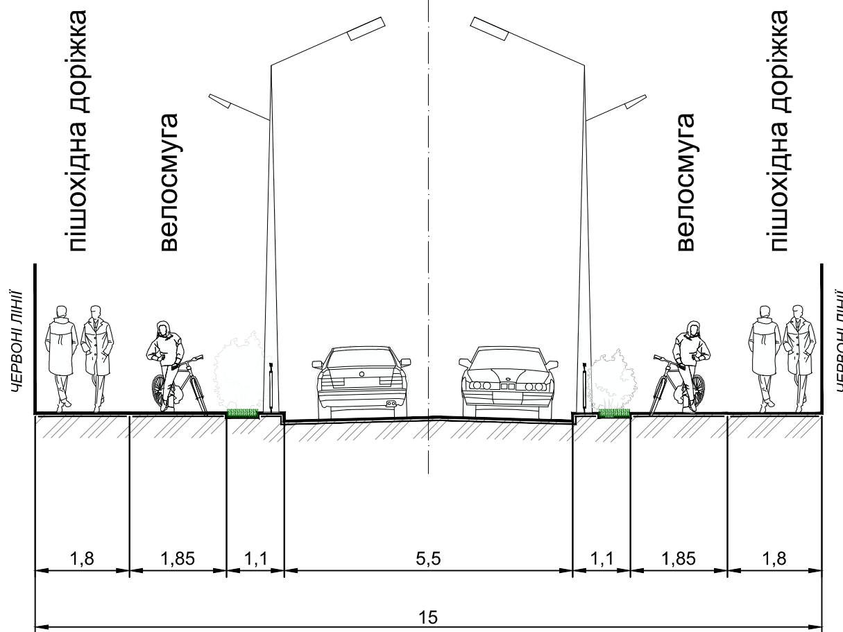
ПРОФІЛЬ 4 - 4 вул. ПРОЄКТНА 53* М 1:100
