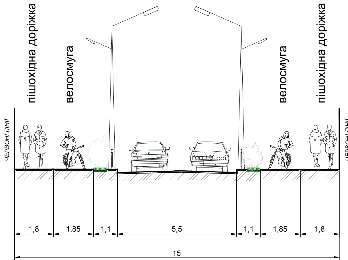
ПРОФІЛЬ 3 - 3 вул. ПРОЄКТНА 48* М 1:100
