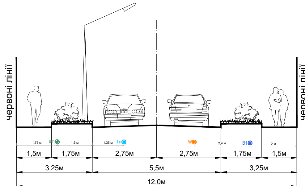
ПРОФІЛЬ І-І
