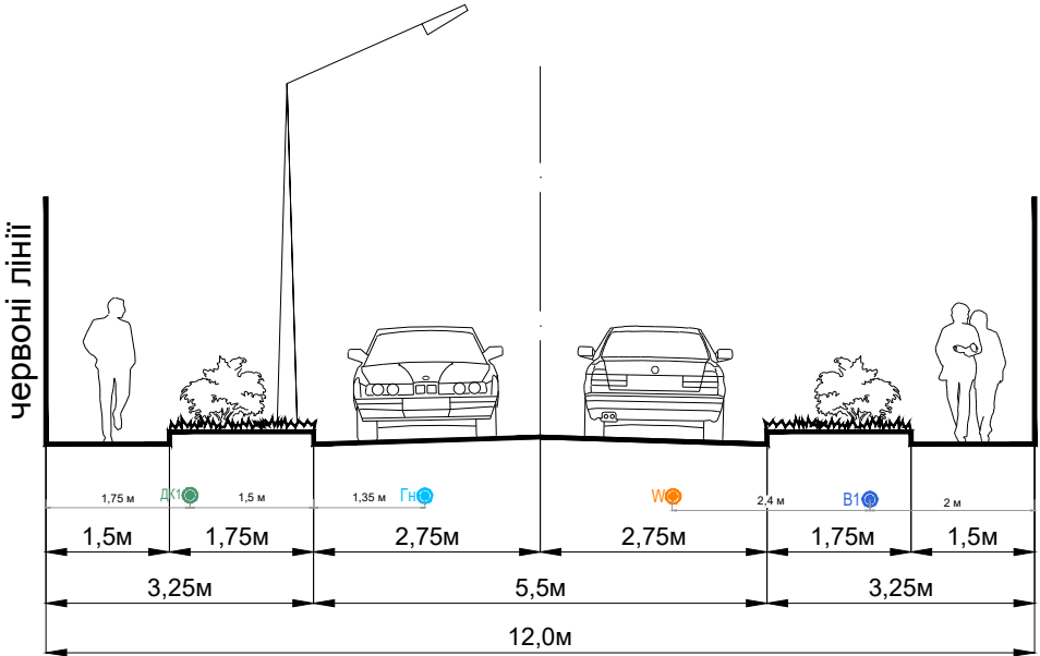
ПРОФІЛЬ І-І
