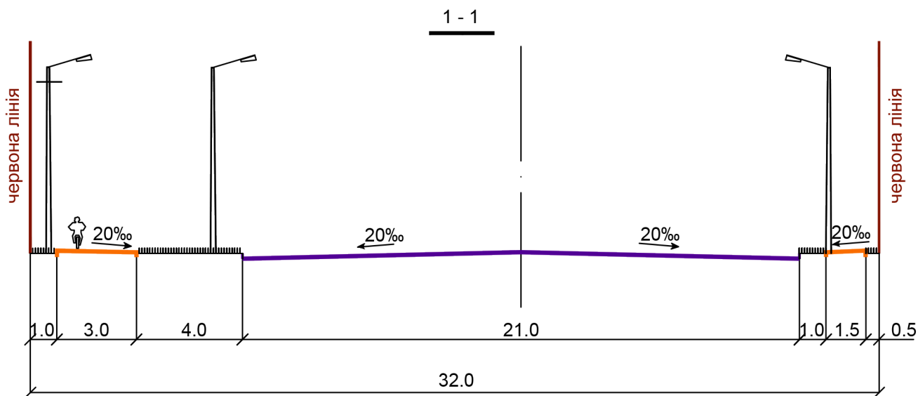
ПОПЕРЕЧНИЙ ПРОФІЛЬ ВУЛИЦІ М1:200
