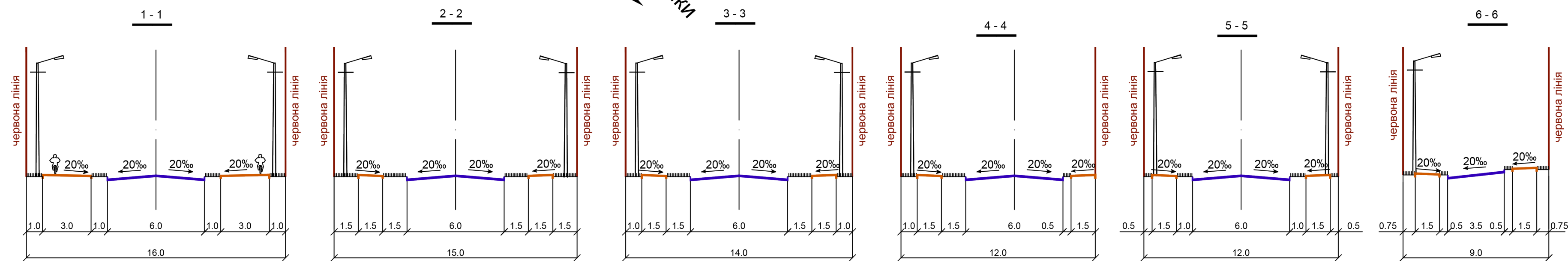
ПОПЕРЕЧНІ ПРОФІЛІ ВУЛИЦЬ M1:200
