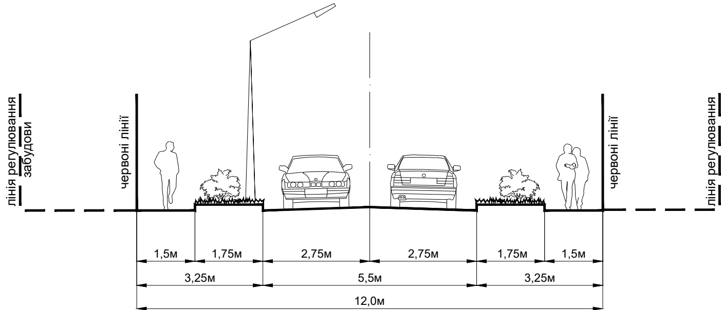
ПРОФІЛЬ І-І
