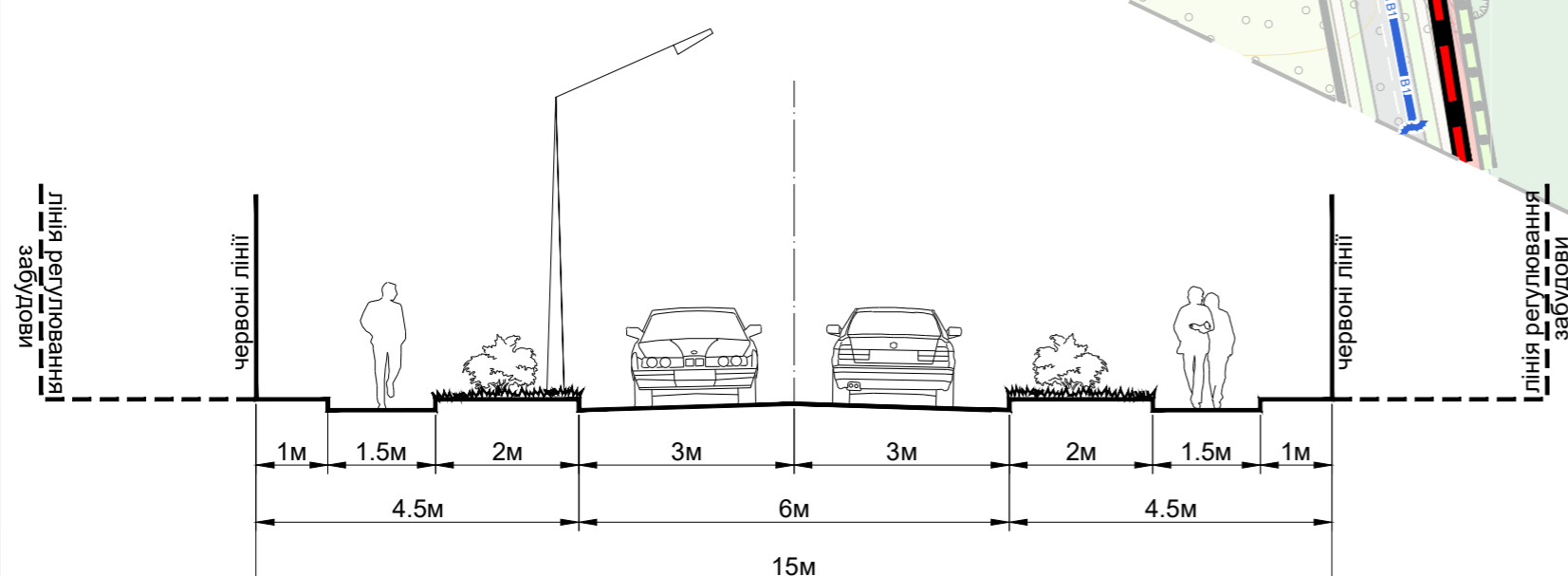
ПОПЕРЕЧНІ ПРОФІЛІ ВУЛИЦЬ, М 1:100: ПРОФІЛЬ І-І
