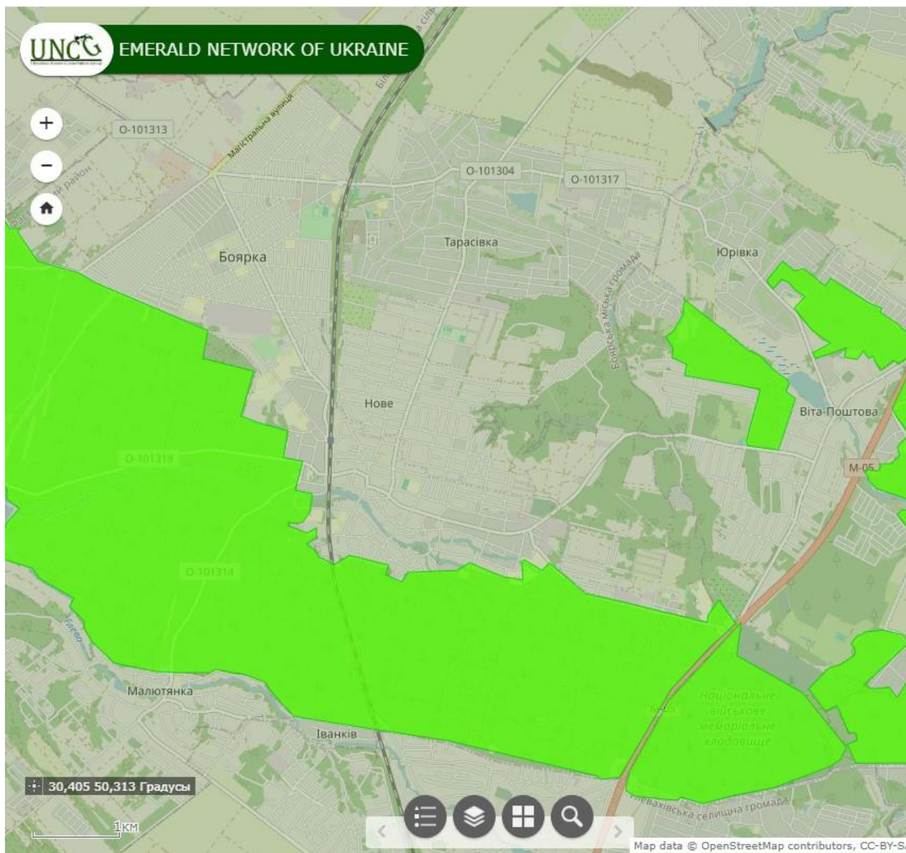
Рисунок 2.1. Об'єкти природно-заповідного фонду в с. Нове Фастівського району Київської області. За даними Emerald Network in Ukraine – Смарагдової мережі України.
