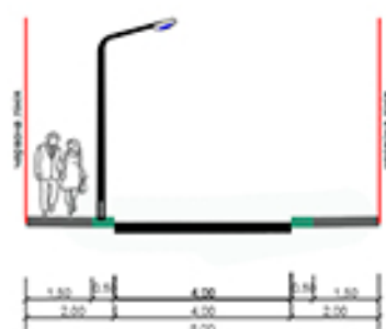
Поперечний профіль вул. І. Миколайчука (проектні рішення)
