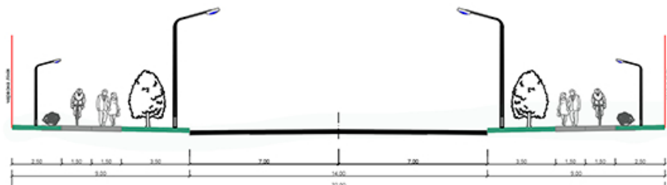
Поперечний профіль вул. Тарасівська (проектні рішення)
