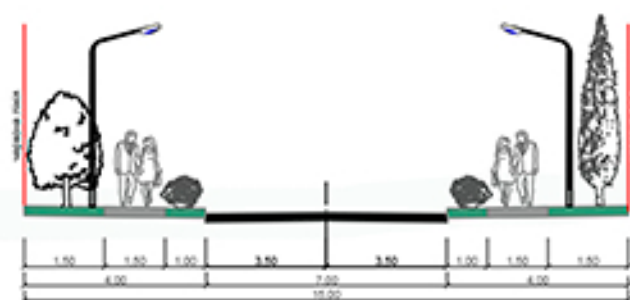
Поперечний профіль інших житлових вулиць
