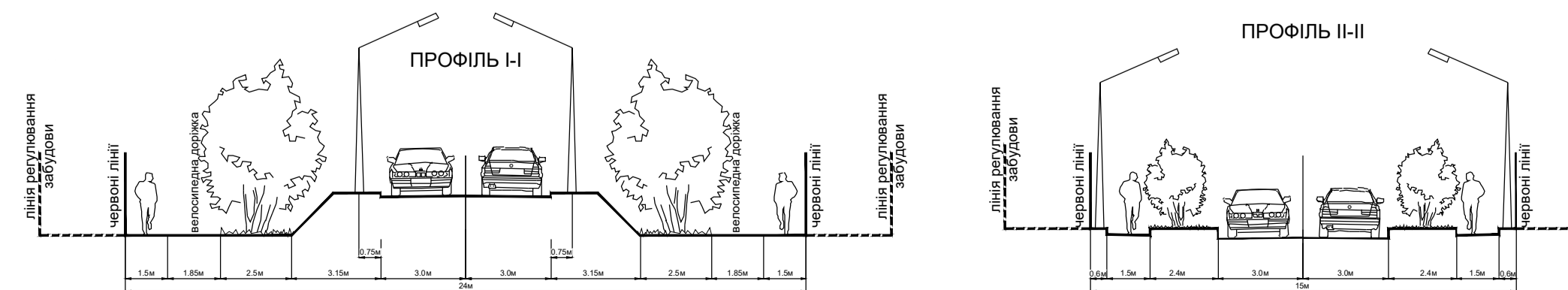
ПОПЕРЕЧНІ ПРОФІЛІ ВУЛИЦЬ М 1:200
