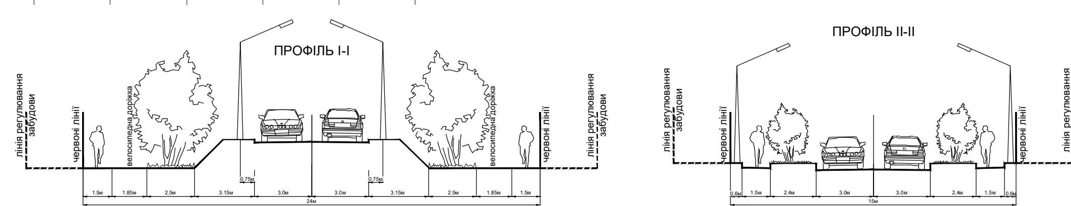
ПОПЕРЕЧНІ ПРОФІЛІ ВУЛИЦЬ М 1:200
